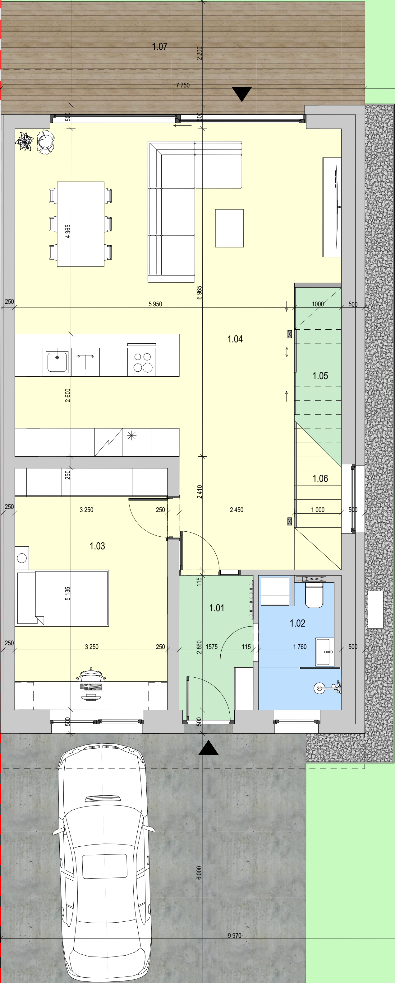
PÔDORYS 1.NP
